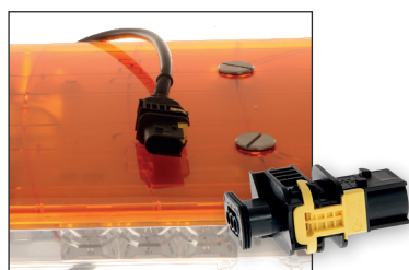
AURUM med 3-polig anslutning till Volvo FH4/FM4/FMX
